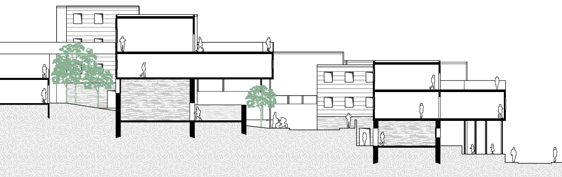
תתך SEC AA המציג את ההתערבות בכפר ההיסטורי
