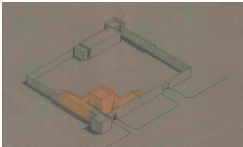
איזומטריה של תחנת נהלל לאחר ההסבה למצודת טיגארט (בכתום מסומן המבנה של תחנת המשטרה האזורית שקדמה לשינוי) מתוך תיק הבניין, ארכיון המדינה
