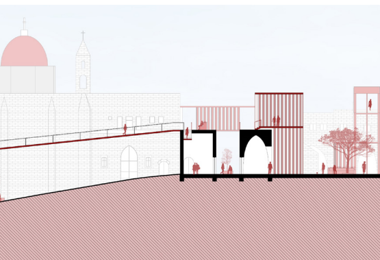
חתך חיבור החיסבא לשוק-סקטור המוסלמים| נקודות החיאה מה
