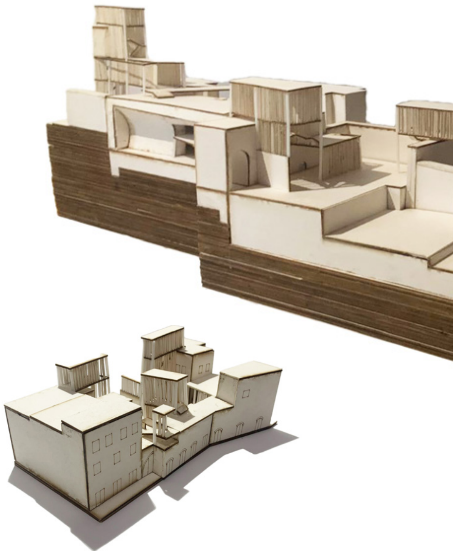
מודל פיזי קנ"מ 1-250 של החצר פנימית בעוגן השוק התלבשות נקודות ההחיא על הגגות
