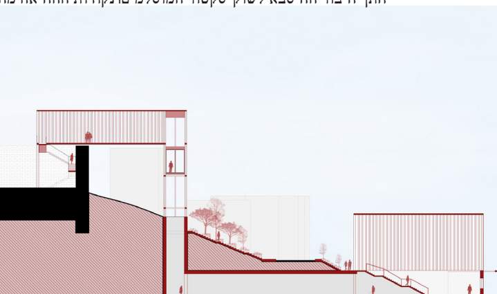
חתך דרך מערכת החיאת המצודה-סקטור הדרוזים| רשת החיאה מחברת את מגדל ה
