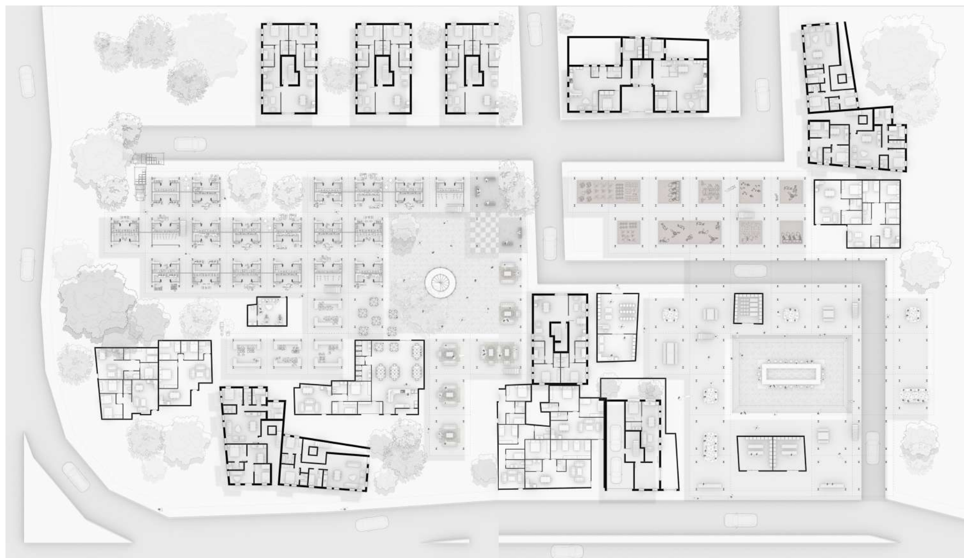
תכנית קומה קרקע
