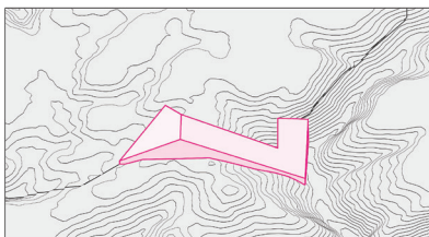
4. קיטום ודירוג כלפי הצד הישראלי
